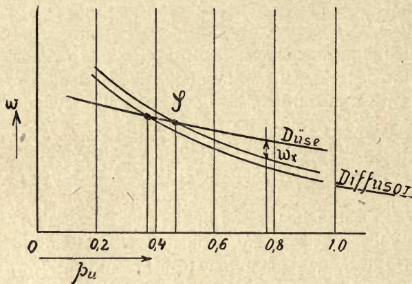
Fig. 3. (Düse = Nozzle).
