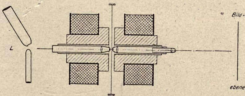
Fig. 8. (Bildebene = Focal plane.)
